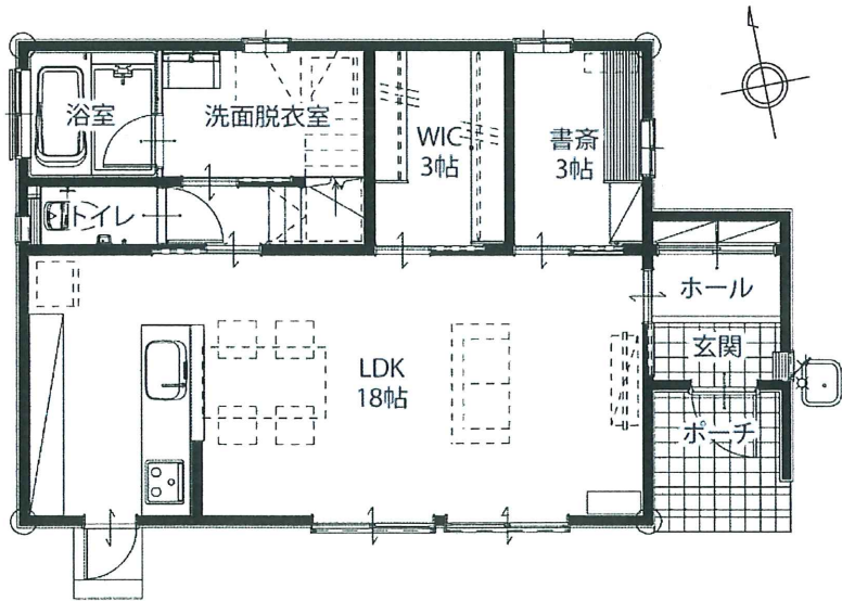
【1階平面図】
